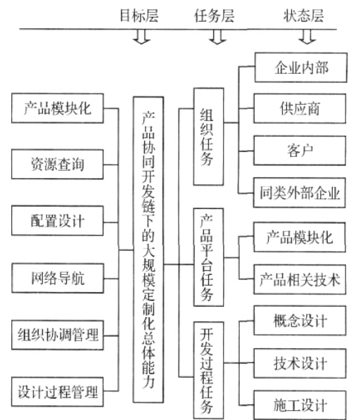
图1 产品协同开发链系统的信息框架
