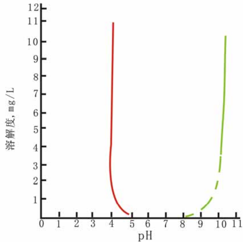
Al 2 O 3 的溶解度与介质pH值的关系 (据科林斯, 1950)
