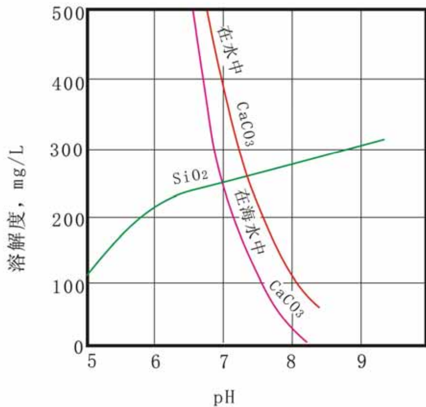
SiO 2 及 CaCO 3 的溶解度与介质pH值的关系 (据科林斯, 1950)
