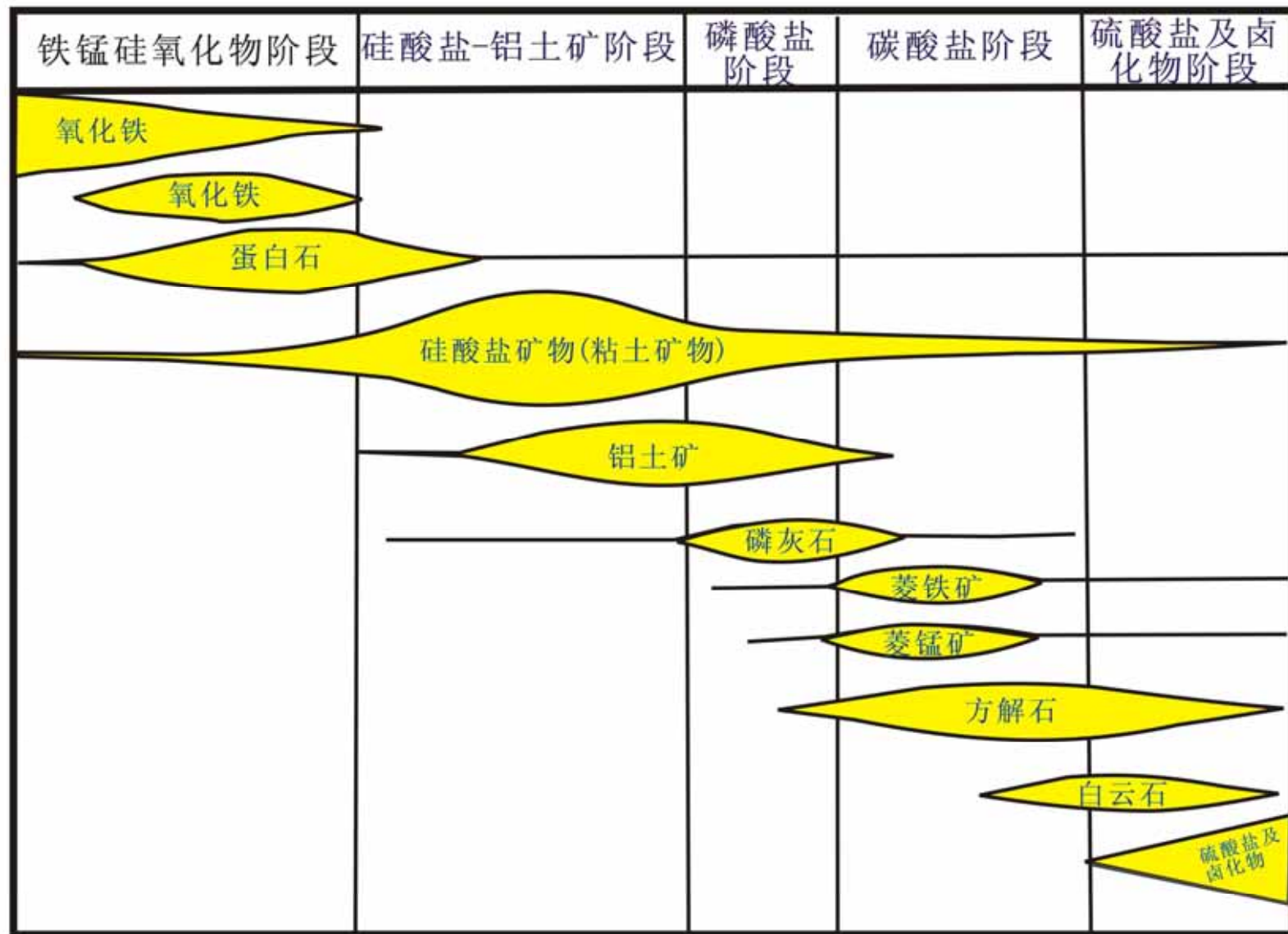
化学沉积分异作用图解(II) (据冯增昭, 1964)
