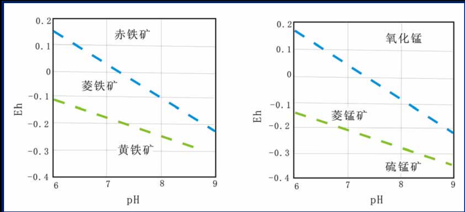
各种铁、锰矿物生成时所需要的pH值及Eh值
