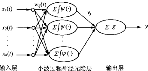
图 2 小波过程神经网络
