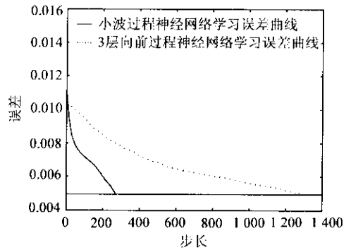
图 3 学习误差曲线
