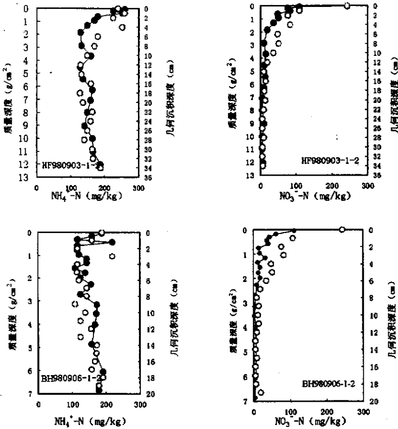
图 3 红枫湖、百花湖沉积物交换性无机氮剖面分布 1 质量深度 ○ 几何沉积深度
