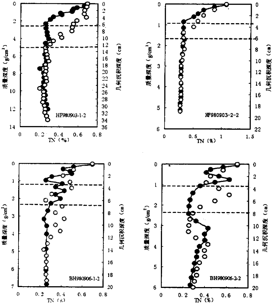
图 1 红枫湖、百花湖沉积物全氮含量剖面分布
