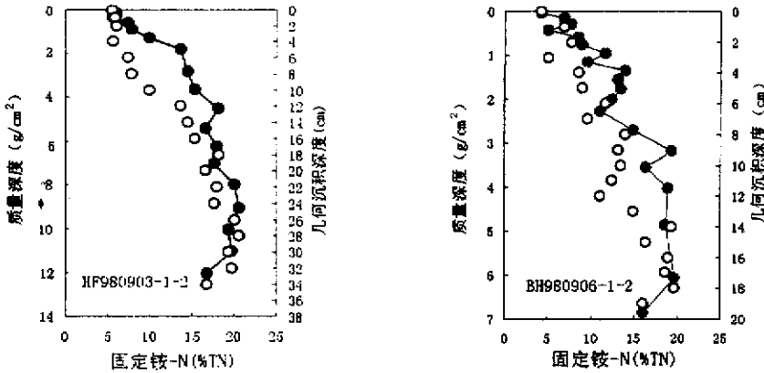
图5 红枫湖、百花湖沉积物固定铵含量相对百分比的剖面分布
