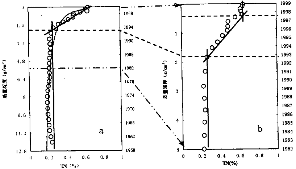
图2 红枫湖 HF980903-1-2 沉积物柱芯全氮降解分析
