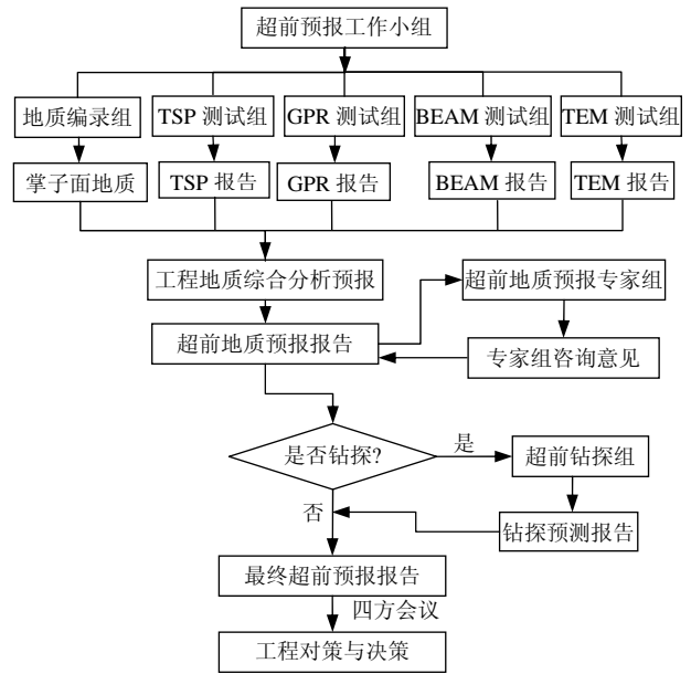
图2 隧道超前地质综合预报组织机构工作流程图
