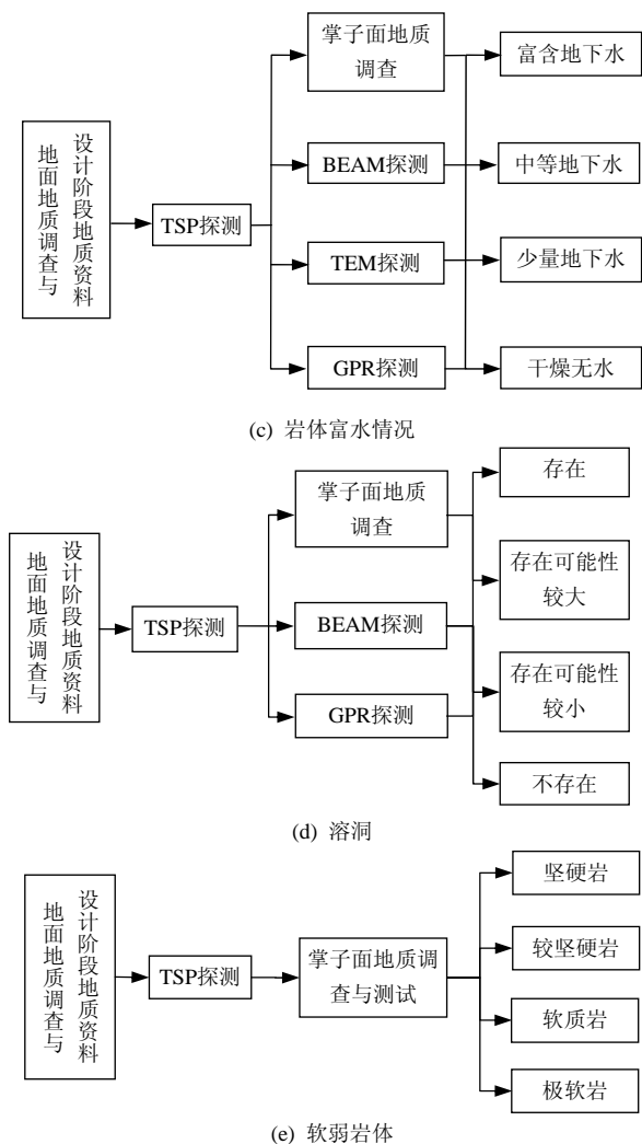
图 3 不良地质条件的综合预报工作方法流程图 Fig.3 Workflow chart of comprehensive prediction for unfavorable geological conditions
