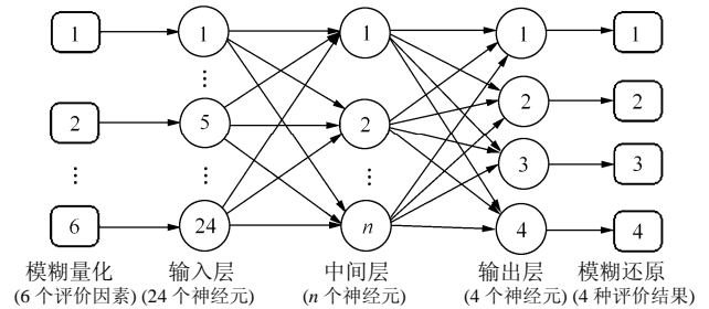
图 4 模糊神经网络结构示意图
