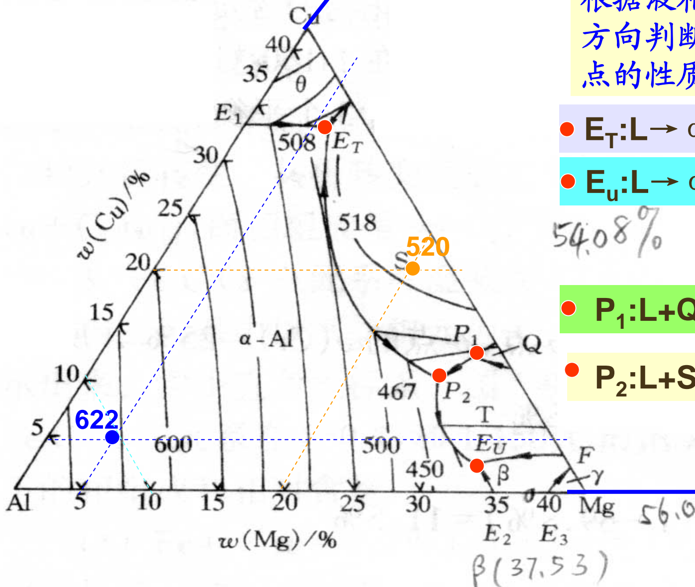
图 5-99 Al-Cu-Mg 三元系液相面投影
