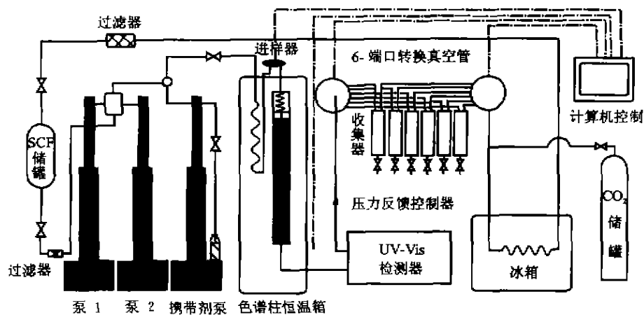
图 1 克级制备型超临界流体色谱示意图
