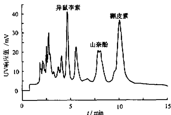
图 2 银杏叶萃取物水解产物的超临界流体色谱分离 YWG-SiO 2 10 \mu\text{m} 柱, 25 MPa, 50 C, 流动相 3.0 mL/min,携带剂为乙醇(其中磷酸体积分数为 0.5%),流动相与携带剂体积比为 90:10
