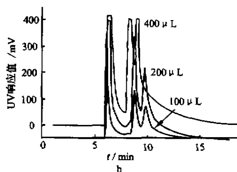
图 3 黄酮、槲皮素、漆树素的分离结果(出峰顺序为黄酮、槲皮素、漆树素)
