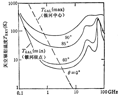
图 4 在 0.1~100GHz 的频率范围内, 几种天顶角下的天空温度的计算值
