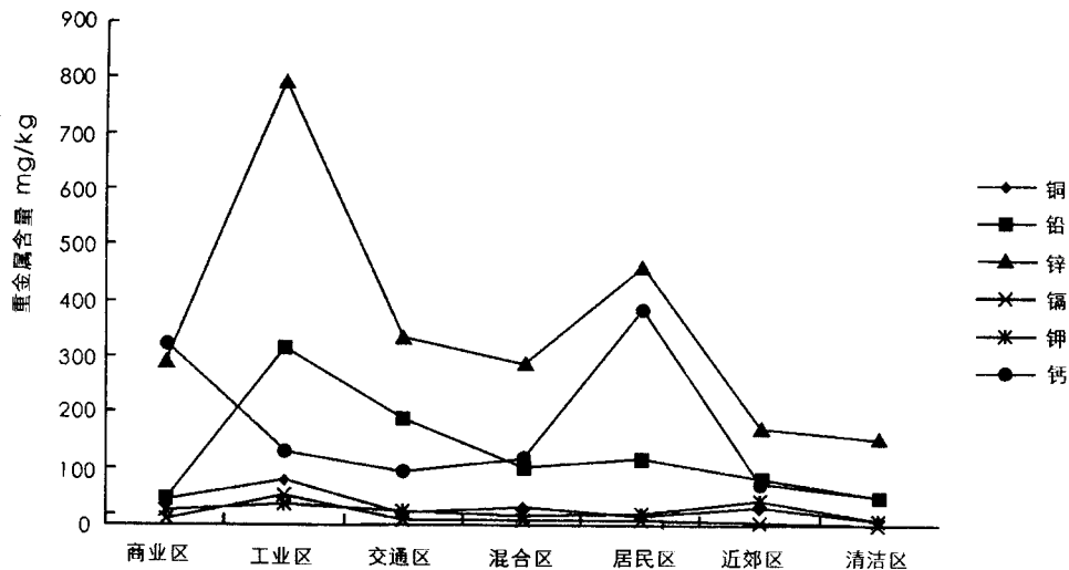
图 2 全市各功能区重金属元素分布曲线
