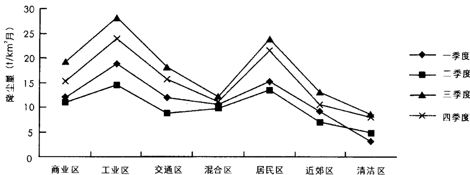
图 1 2004年全市各功能区大气降尘季节分布曲线
