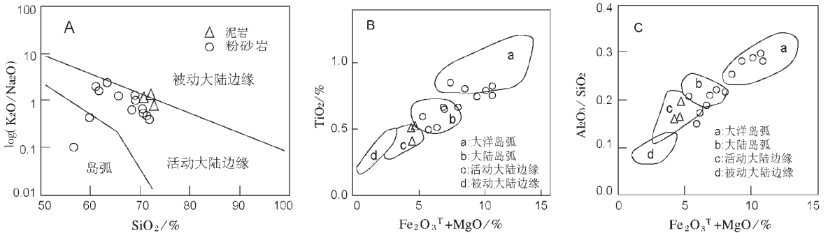
图6 砂岩形成构造环境判别图
