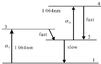
图1 Cr离子能级结构图
