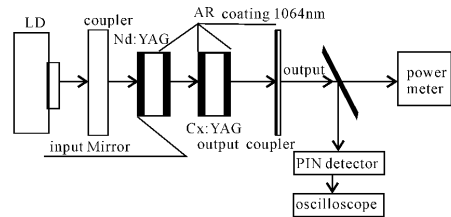
图2 被动调Q激光器实验装置示意图
