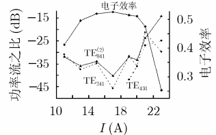
图 10 杂模功率流(相对于 TE_{04} 模基波分量)及电子效率随电流的变化
