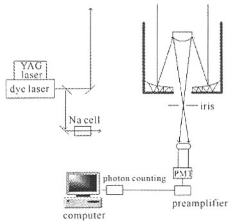
Fig. 1 Schematic diagram of Na fluorescence lidar 图 1 钠荧光激光雷达原理示意图
