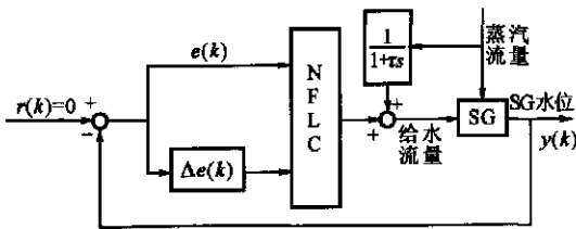
图4 模糊神经网络水位控制器 [19]
