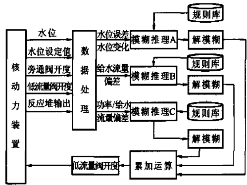
2 Fugen 堆 SG 水位模糊控制推理框图(低流量) [17]
