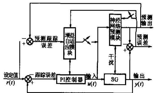
图 3 SG 水位神经网络预测控制 [18]
