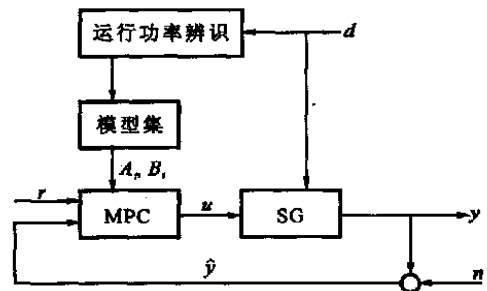
图 1 SG 水位模型预测控制
