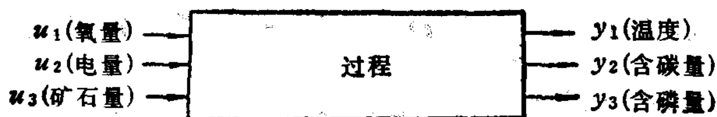
图 1 氧化期冶炼过程简化框图
