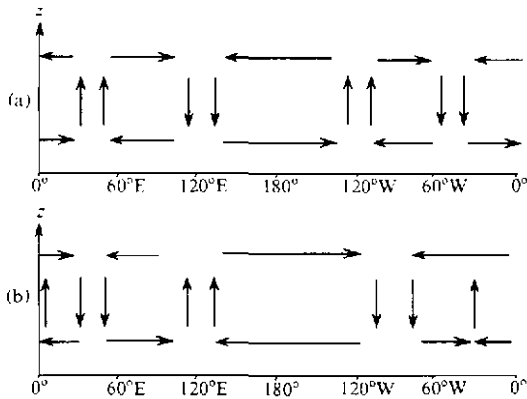
图 7 与赤道印度洋海温偶极子正位相 (a) 和负位相 (b) 相对应的赤道大气的异常纬向垂直环流特征示意图
