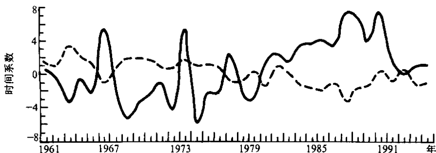
图3 由SVD得到的右场1960~1993年1~10月青藏高原地面加热强度场与左场1961~1994年1~4月高原上空100 hPa高度场第一模态的时间系数 T_1 (虚线) T_{12} (实线)
