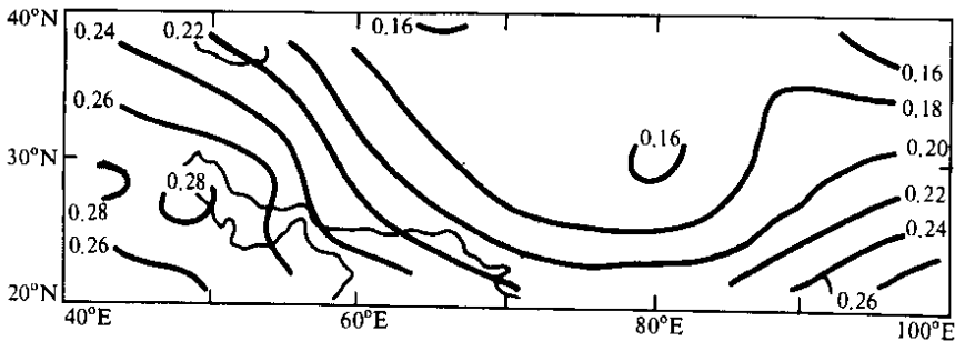
图 2 由 1960~1993 年 1~10 月青藏高原地面加热强度场与 1961~1994 年 1~4 月高原上空 100 hPa 高度场 SVD 得到的左场 100 hPa 高度场第一模态的空间结构
