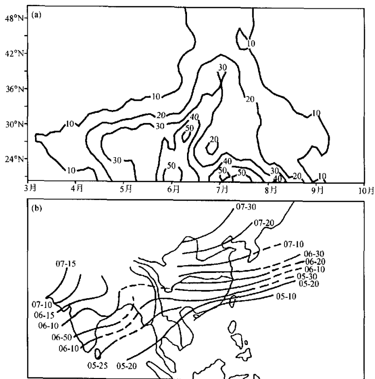
图2 (a) 东亚地区 1961~2000 年平均的沿 115°E (110°~120°平均) 5 天降水量的纬度—时间剖面图 (单位: mm); (b) 东亚夏季风暴的平均日期 (引自文献 [20])
