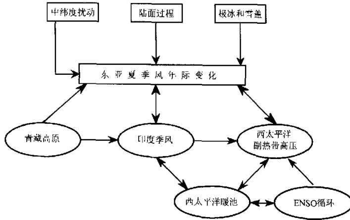
图 5 影响东亚夏季风年际变化的物理因子示意图
