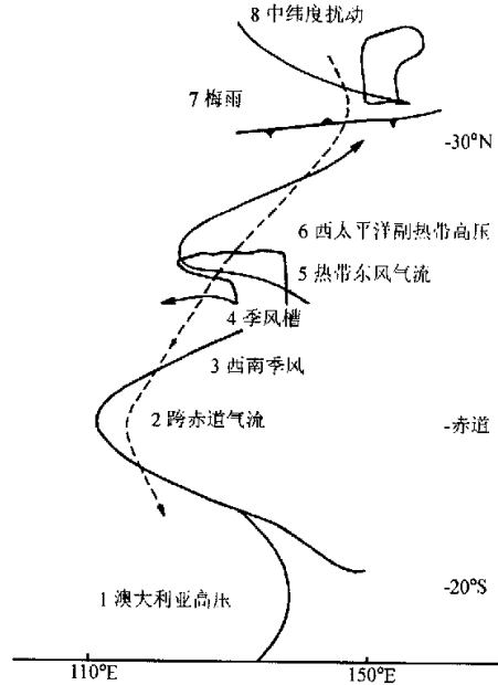
图1 东亚夏季风系统成员的配置(引自文献[20])
