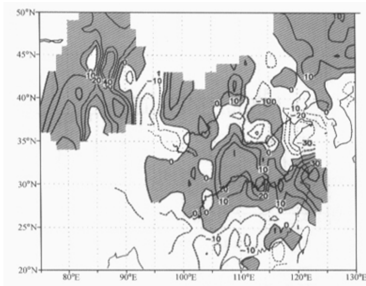
图 6 中国 1977~2000 年与 1967~1976 年夏季 (6~8 月) 平均降水距平百分率之差 阴影区为正值, 虚线区为负值
