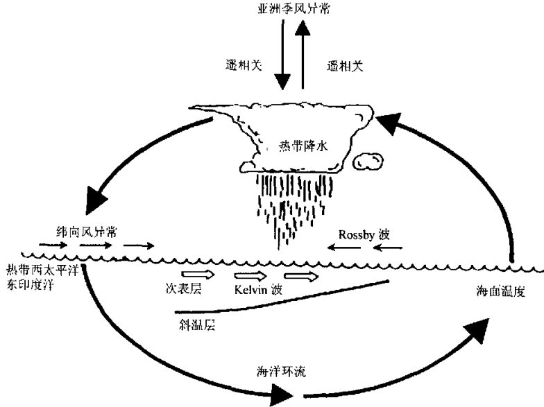
图 9 亚洲季风与 ENSO 循环相互作用过程示意图
