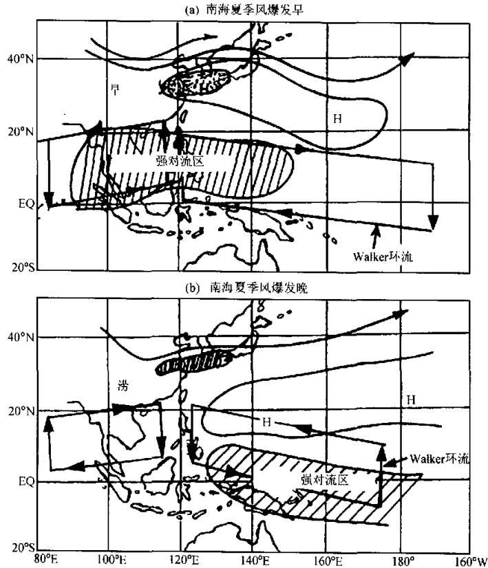
图3 西太平洋暖池热状况、西太平洋副热带高压、南海季风爆发日期之间的关系
