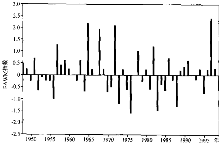
图 7 1951~2000 年东亚冬季风指数的年际变化
