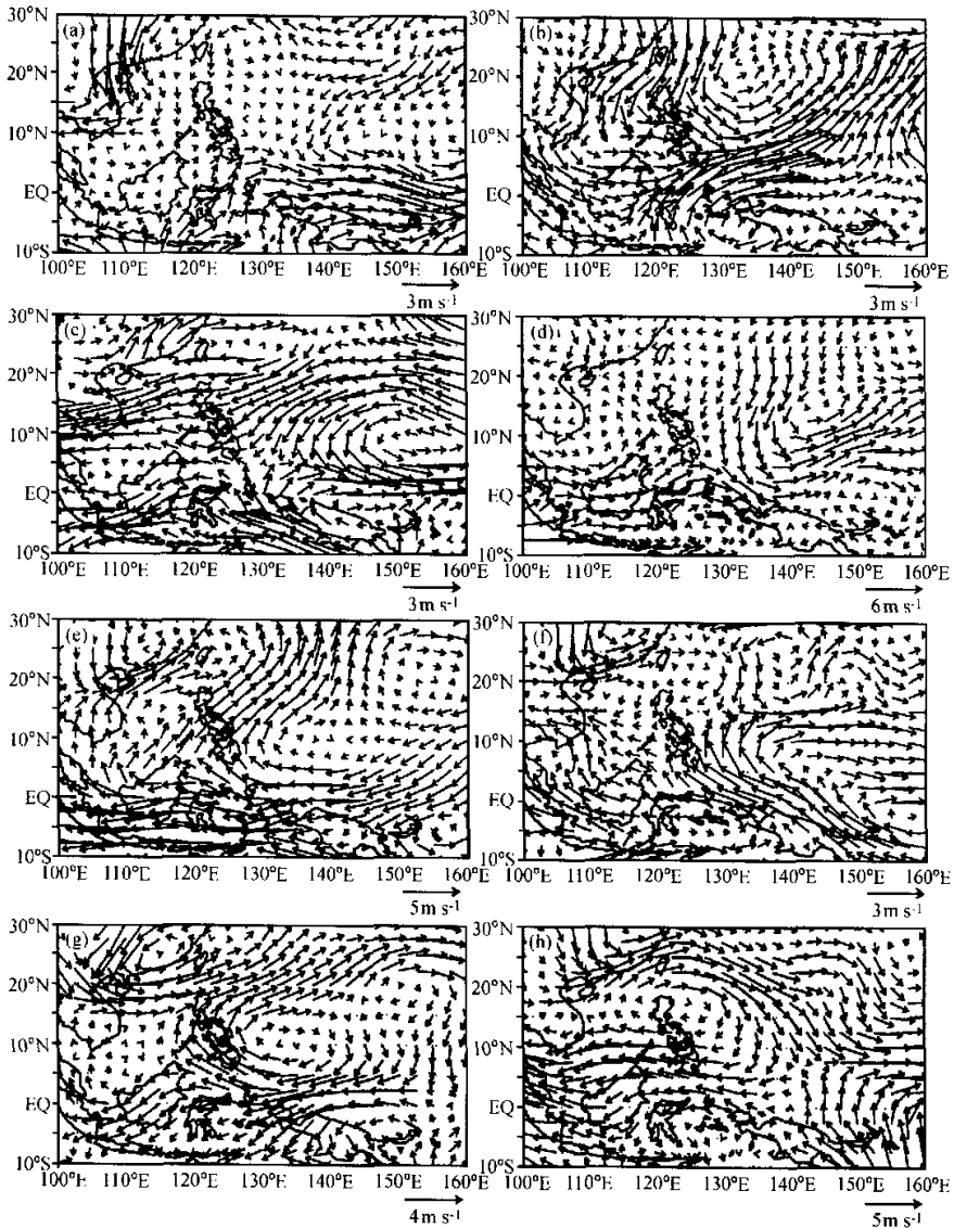
图 8 1980~1998 年 4 次 El Niño 事件发展阶段 (a~d) 以及成熟阶段 (e~h) 时热带西太平洋上空 850 hPa 距平风场分布
