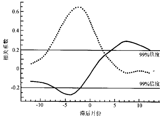
图 10 西太平洋暖池次表层 (120~160m) 异常海温东传与赤道西太平洋异常纬向风 (虚线) 以及西北太平洋地区异常经向风 (实线) 的时滞相关系数随时间的演变 (引自文献 [77]), 负值表示异常海温东传超前
