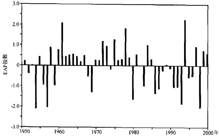
图 4 1951~2000 年夏季 EAP 指数的年际变化 (引自文献 [28])
