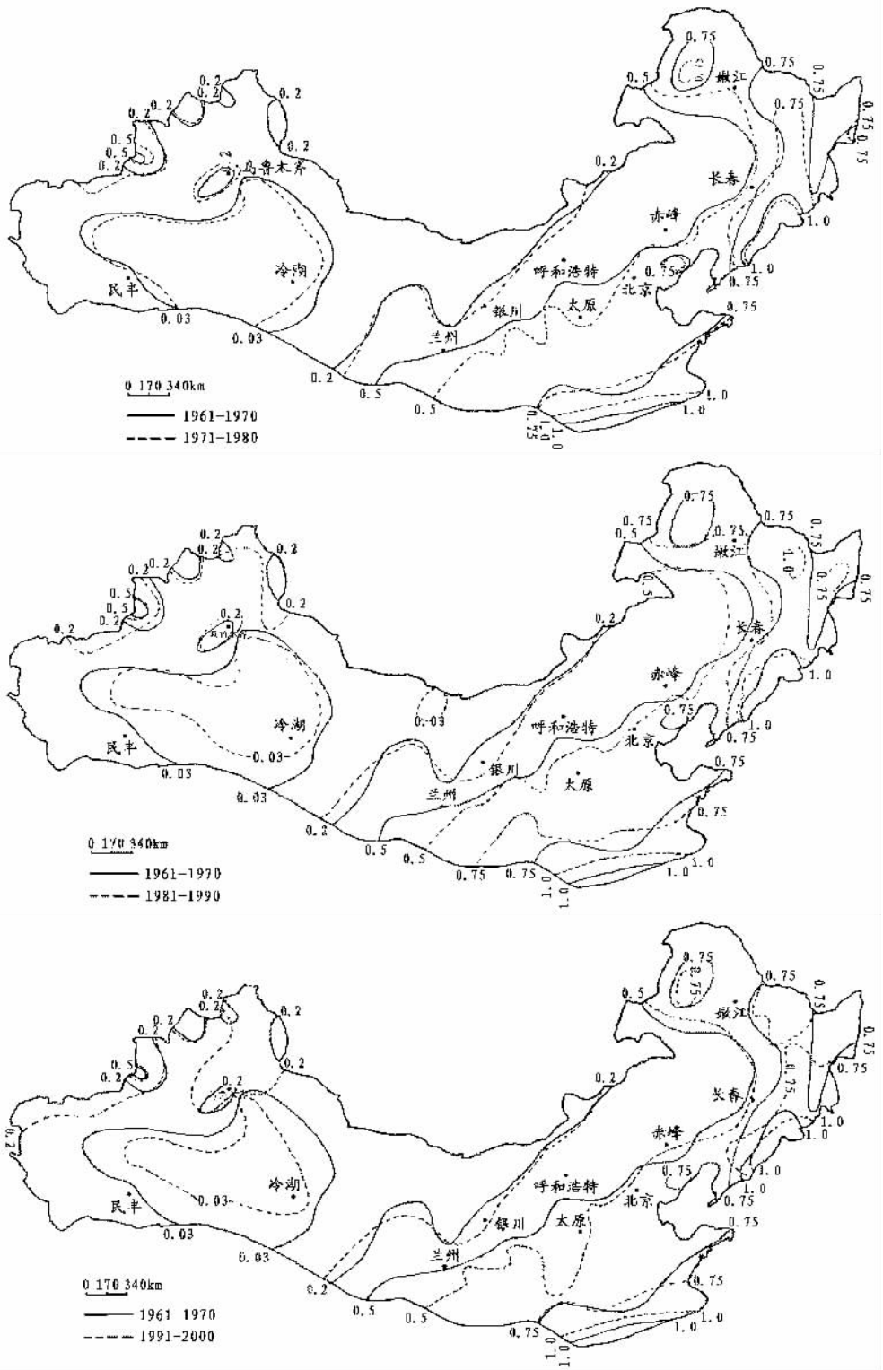
图 2 气候干湿带 10 年际变化
