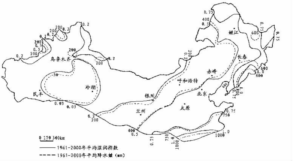
图 1 中国北方干湿气候带与降水量分布图
