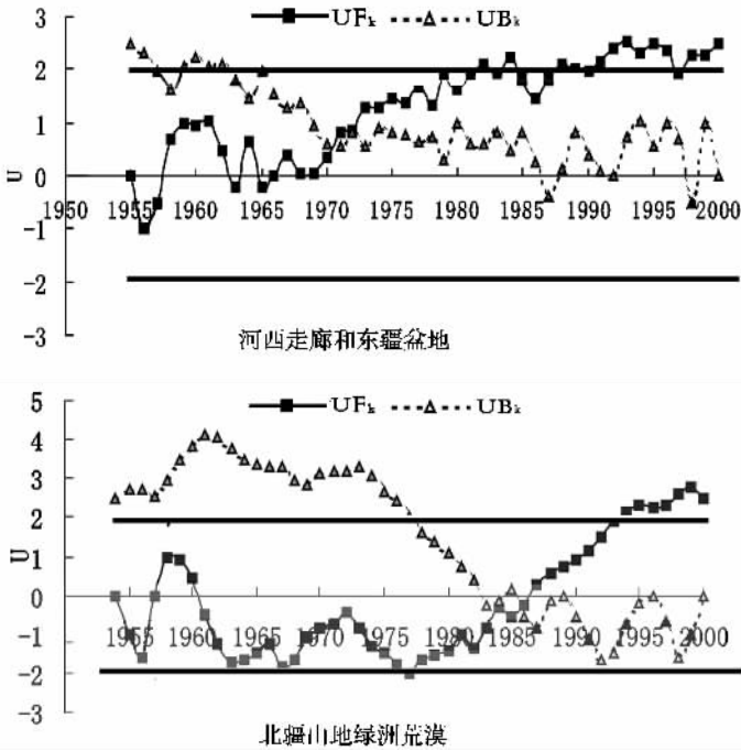
图 3 湿润指数 Mann-Kendall 统计量曲线 (直线为 \alpha=0.05 显著性水平临界线)
