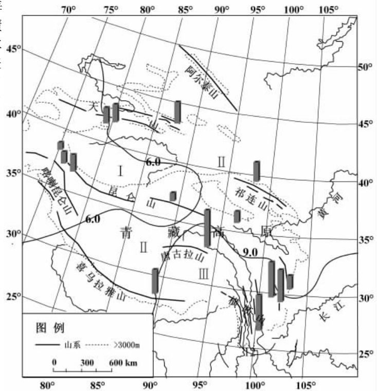
图 4 中国西部度日因子变化趋势及其分区(图中柱状代表度日因子值),其中 I 为 DDF 低值区( \leq 6.0 \text{ mm d}^{-1} \text{ }^{\circ}\text{C}^{-1} ), II 为 DDF 中值区( 6.0\sim 9.0 \text{ mm d}^{-1} \text{ }^{\circ}\text{C}^{-1} ), III 为 DDF 高值区( \geq 9.0 \text{ mm d}^{-1} \text{ }^{\circ}\text{C}^{-1} )
