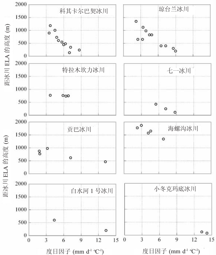
图 2 中国西部冰川度日因子随距冰川 ELA 距离的减小而增大
