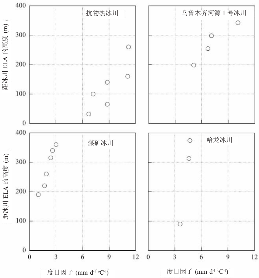
图 3 中国西部冰川度日因子随距冰川 ELA 距离的减小而减小。
