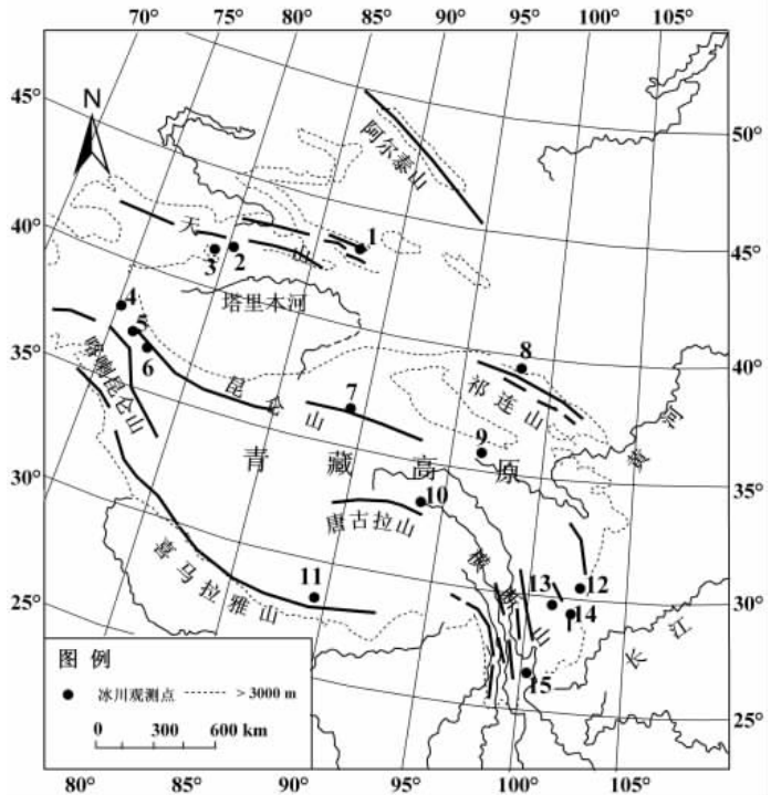
图1 中国西部观测冰川分布图。
