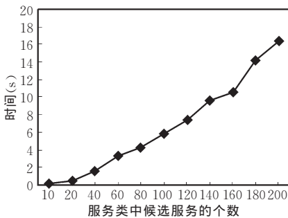
图 2 服务类中候选服务的个数与服务查找时间之间的关系
