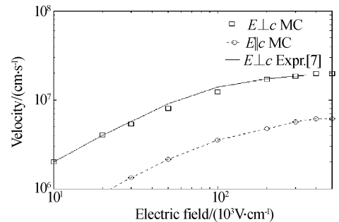
图 2 296 K 时,电子漂移速度随电场的变化
