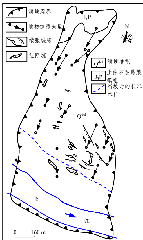
图4 鸡扒子滑坡平面图 [43]
