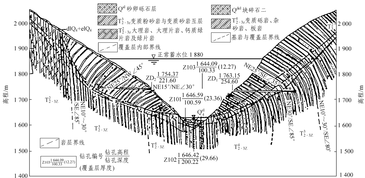
图 21 雅砻江水文站坝址剖面工程地质剖面图 [56] (单位: m)
