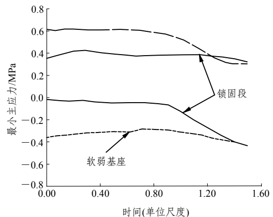
图 18 最小主应力与时间的关系曲线
