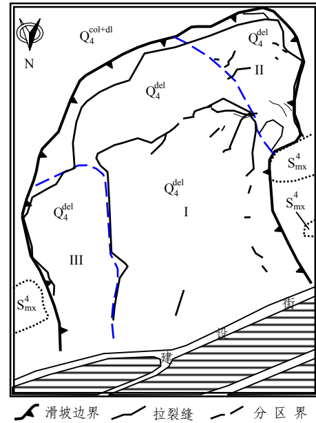
图 14 丹巴滑坡工程地质略图
