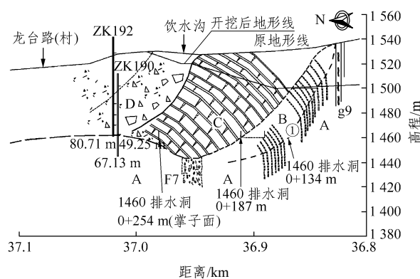
A—直立岩体; B—倾倒松弛岩体; C—(倾倒)坠伏堆积; D—(崩)堆积; ①—最大弯曲折断面
