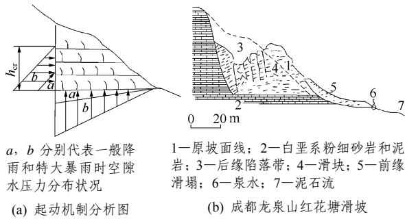
图 20 特大暴雨条件下产生的平推式滑坡 [45]
