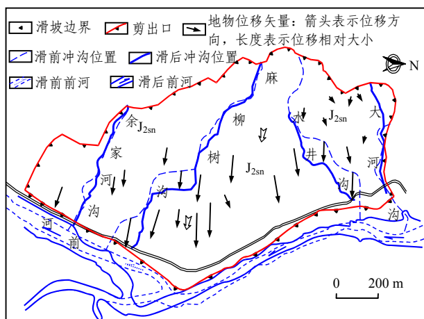
图11 天台乡滑坡工程地质平面略图
