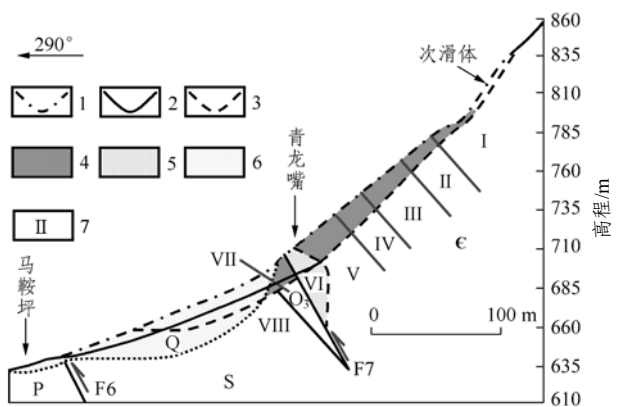
1—初始地形线；2—滑后地形线；3—滑动面；4—强风化带；5—钙质角砾岩；6—第四系崩塌堆积物；7—岩体结构分区(I：层块碎裂结构；II：厚层状结构；III：层状结构；IV：层状碎裂结构；V：碎裂结构；VI：角砾状结构；VII：奥陶系层状灰岩；VIII：志留系泥、页岩)；c—寒武系地层；S—志留系地层；P—二迭系地层；Q—第四系地层
