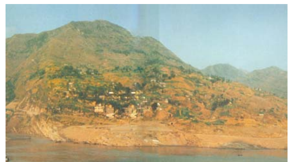
图 3 长江鸡扒子滑坡(1982 年) Fig.3 Jipazi landslide on Yangtze River in 1982
