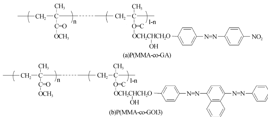
图 1 偶氮苯聚合物分子结构式
