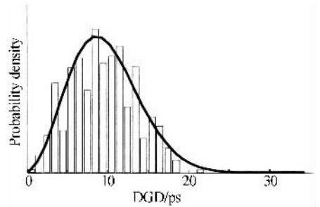
图 3 模拟器 DGD 测量值的统计结果
