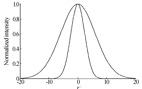
图 4 反射镜上荧光与激光的归一化强度分布
