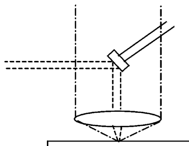
图 2 几何光束分离器示意图 Fig. 2 Schematic diagram of geometric beamsplitter
