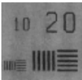
图 6 10 \mu\text{m} 分辨率扫描图
