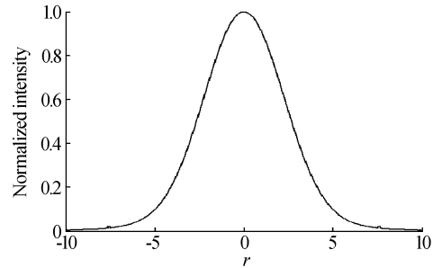
图 3 生物芯片上激光强度分布
