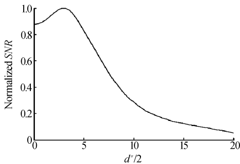
图 5 随反射镜孔半径的 SNR 变化曲线
