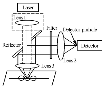
图 1 实验原理图 Fig. 1 Schematic diagram of the experiment
