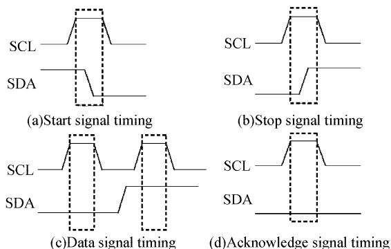
图 2 信号时序图
