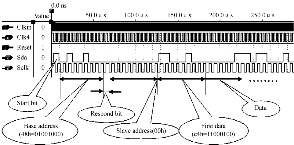
图 5 I2C 总线仿真波形
