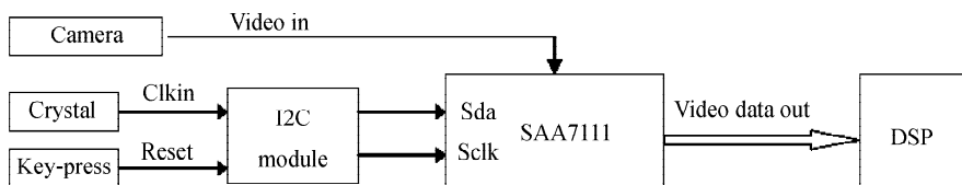
图 1 系统功能框图
