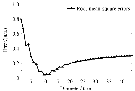
图3 测量所得散射光强角分布与理论值的根均方差
