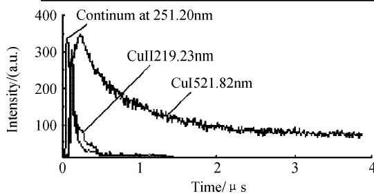
图 3 在 25.7 kPa 的 Ar 气下, 离靶 0.6 mm 处的 Cu 背景光谱线的强度随时间的分布
