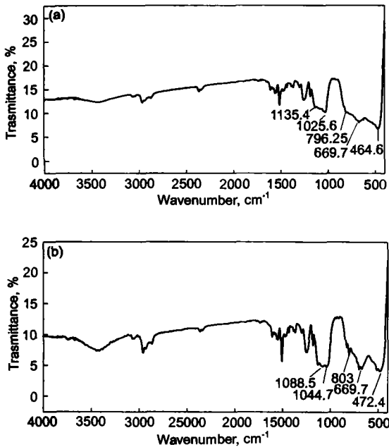
图7 AO 辐照 TiO 2 -有机硅涂层前后的 FTIR 谱
