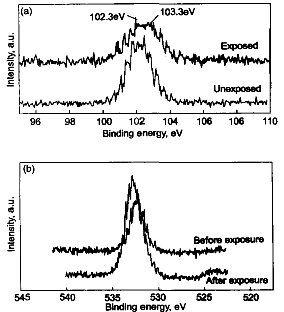
图 6 TiO 2 -有机硅涂层暴露 AO 环境前、后的 XPS 图
