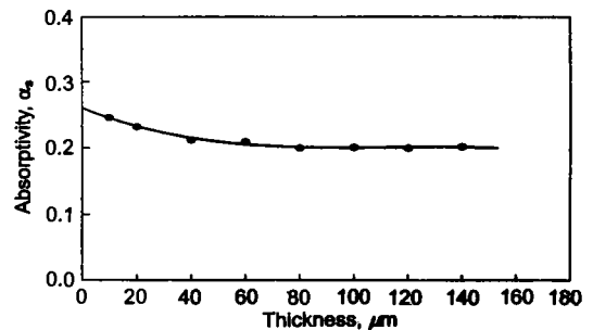
图 1 涂层厚度对 α s 的影响
