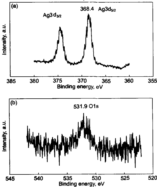
图 5 AO 辐照后 Ag 试样表面的 XPS 图
