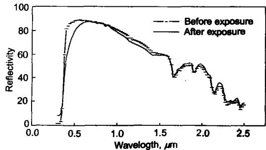
图 4 TiO 2 -有机硅涂层的光谱反射率
