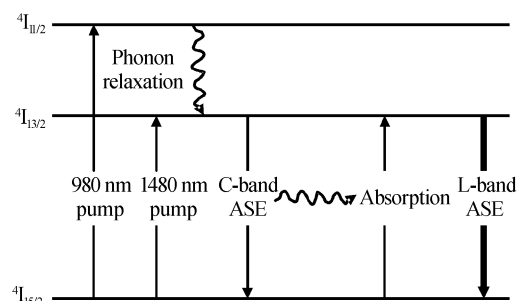
图 1 铒离子能级
