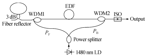
图 2 双程双向泵浦的 L 波段 ASE 光源结构 Fig. 2 Schematic diagram of the DP-BD pumped L-band ASE source
