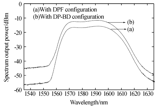
图 3 输出 L 波段 ASE 谱 Fig. 3 Output L-band ASE spectrum
