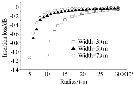
图 3 宽度不同的弯曲波导, 曲率半径与插入损耗的关系图 Fig. 3 The relationship of radius and insertion loss for varying bend widths
