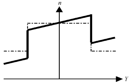
图 1 弯曲波导截面的折射率分布
