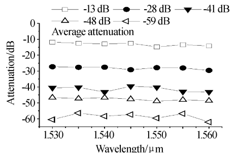
图 6 VOA 在不同衰减水平上的波长敏感度
