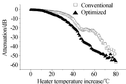
图 4 优化电极位置前后 VOA 衰减曲线的比较
