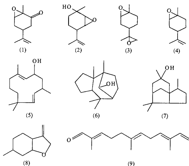
图 1 PI312777 土培的根系分泌物乙醚萃取物中萜类化合物结构 Fig.1 Terpenoids of ether extracts from the PI312777 root exudates grown in soil.
