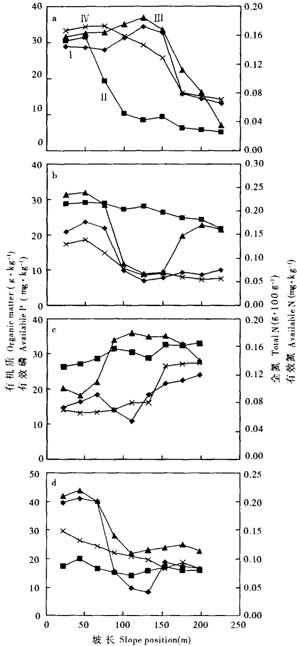
图 1 不同土地利用方式下土壤营养元素的分布 Fig. 1 Distribution of soil nutrients under different land use type. a) 草地-耕地-林地 Grassland-cropland-woodland; b) 林地-耕地-草地 Woodland-cropland-grassland; c) 耕地-草地-林地 Cropland-grassland- woodland; d) 人工草地-天然草地-林地 Cultivated grassland-grassland- woodland. I. 有机质 Organic matter; II. 全氮 Total N; III. 有效氮 Available N; IV. 有效磷 Available P. 下同 The same below.
