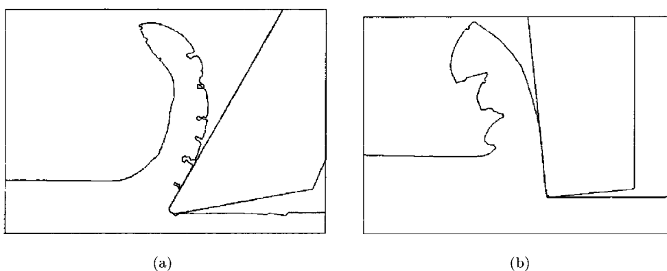
图 7 切屑断裂时的模拟结果
