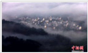
安徽齐云山现平流云海景观
