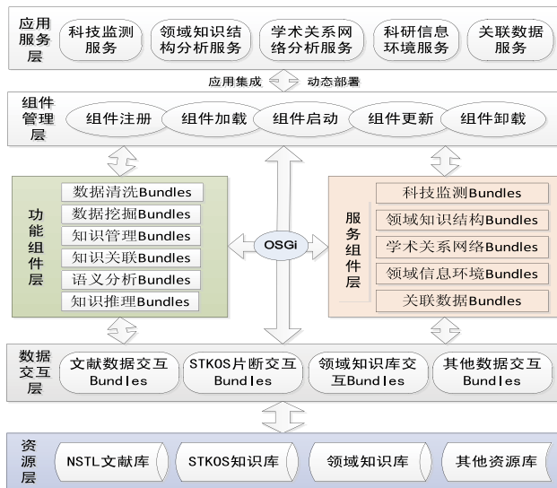
图1 基于OSGi的知识服务应用示范系统体系架构
