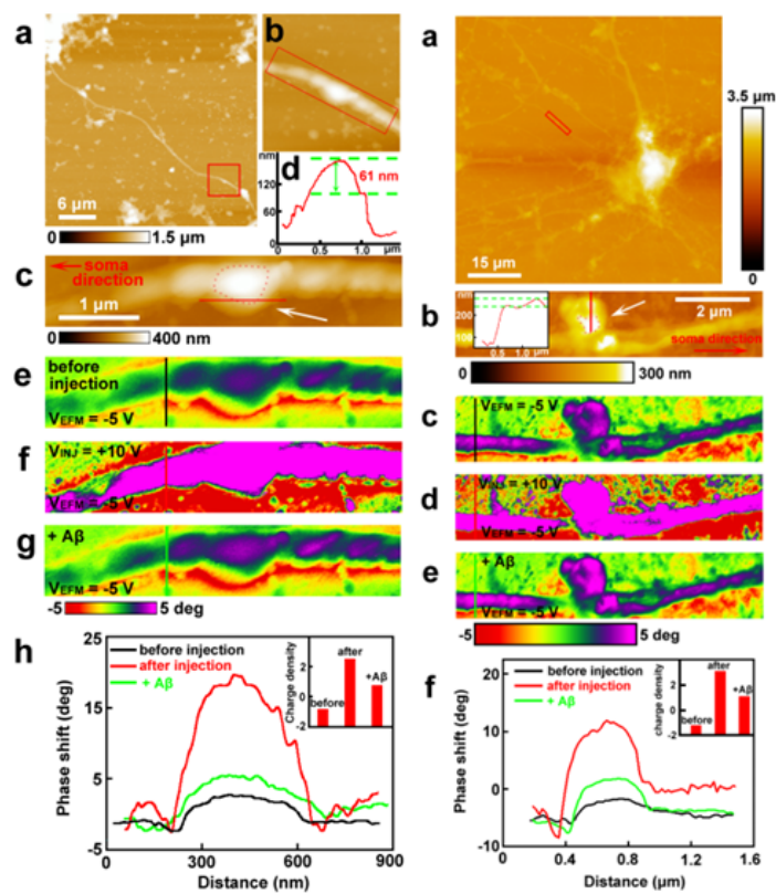
图2 静电显微镜分别研究电荷在轴突（左图）和树突（右图）中的传递
