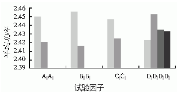
图7 正交试验因素水平与平均电功率的关系
