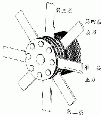
图1 刀片的安装
