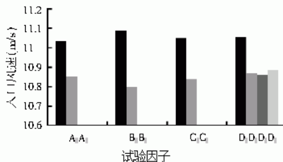
图6 正交试验因素水平与入口风速之间的关系
