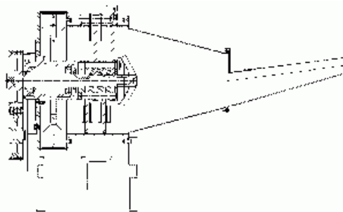
图2 9RZ-60型秸秆揉切机结构
