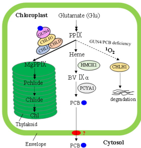
图1 叶绿体信号分子胆色素(PCB)和GUN4调控叶绿素合成的模式图
