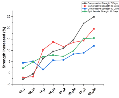
图1 预处理橡胶混凝土强度
