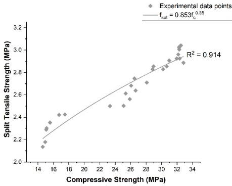
图2 抗压和劈裂抗拉强度关系式
