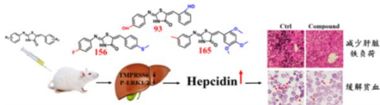
图1. 噻唑烷酮类化合物增加Hepcidin表达来阻止铁负荷与改善贫血
