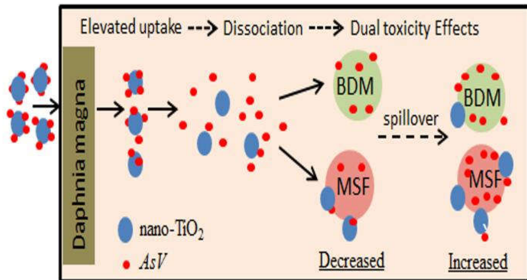
纳米二氧化钛对大型蚤五价砷的生物可利用性及毒性效应的影响概念图
