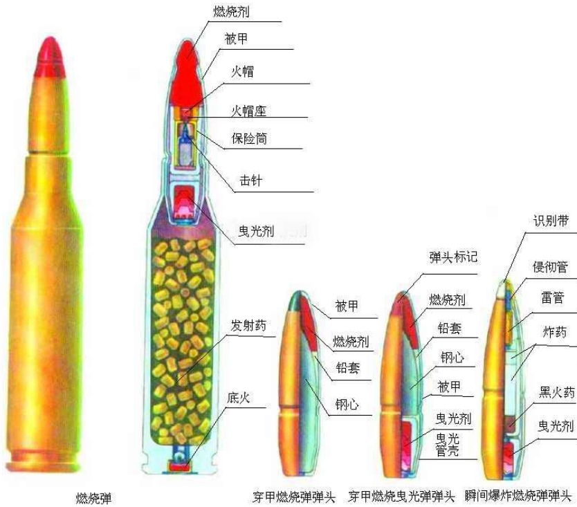
燃烧弹 穿甲燃烧弹弹头 穿甲燃烧曳光弹弹头 瞬间爆炸燃烧弹弹头剖视图
