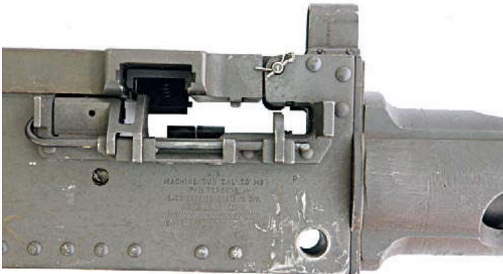
6 拉机柄与枪机采用分离式设计，向后拉动拉机柄，通过连接在枪机上的枪机驻笋带动枪机向后运动。该枪机匣两侧均加工有拉机柄导槽，因此拉机柄可根据需要装在机匣的任一侧
