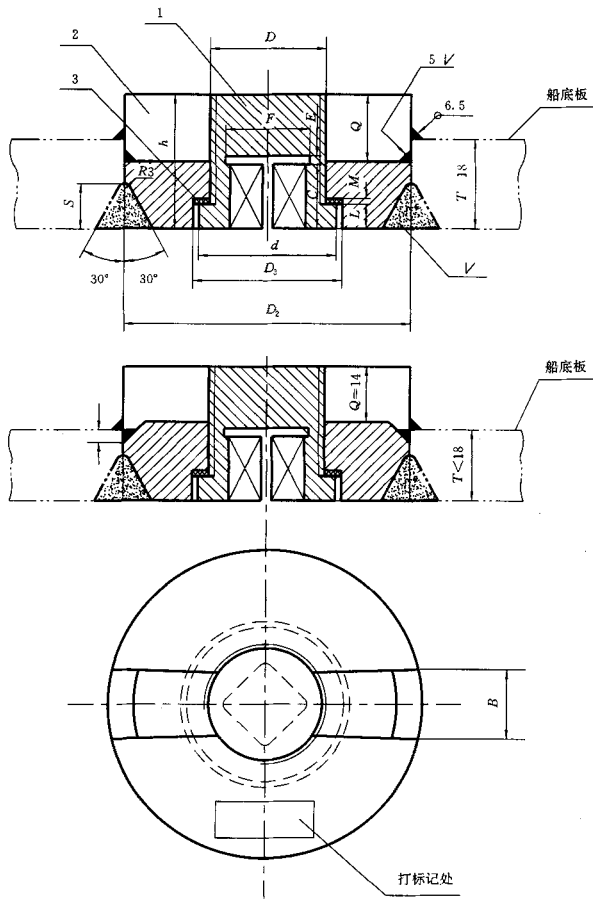
图 1 A 型螺塞
