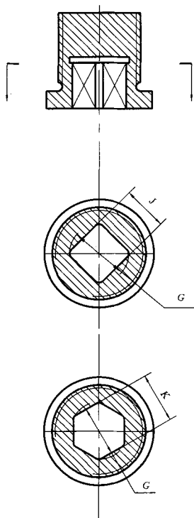
图 3 旋塞
