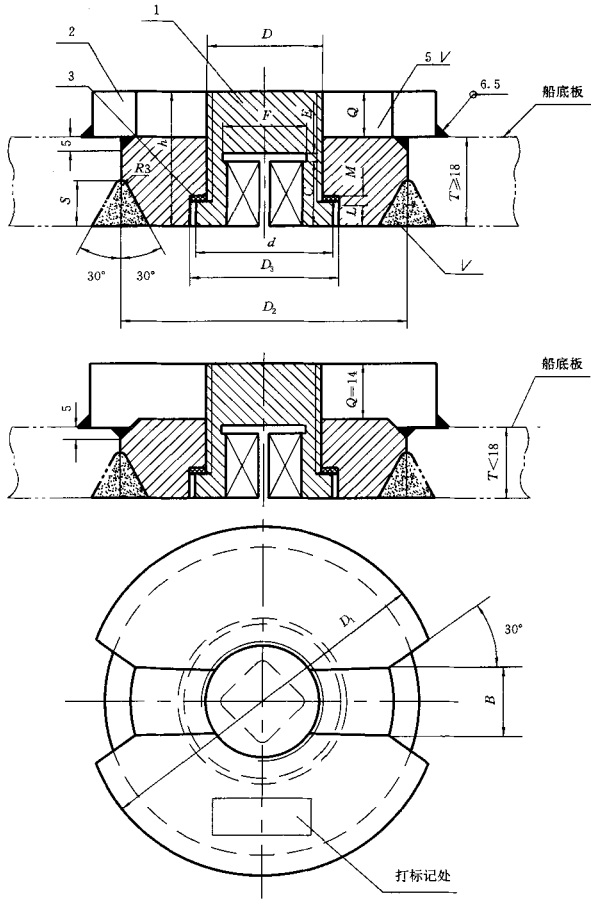
图2 B型螺塞
