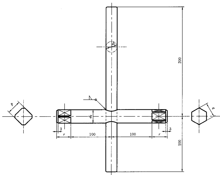
图 4 扳手 表 3 扳手尺寸
