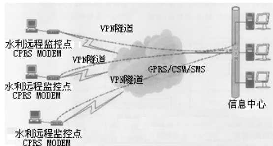
图1 智能水利远程监控系统网络结构图
