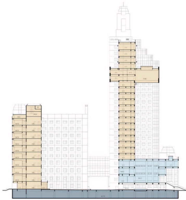
剖面图
