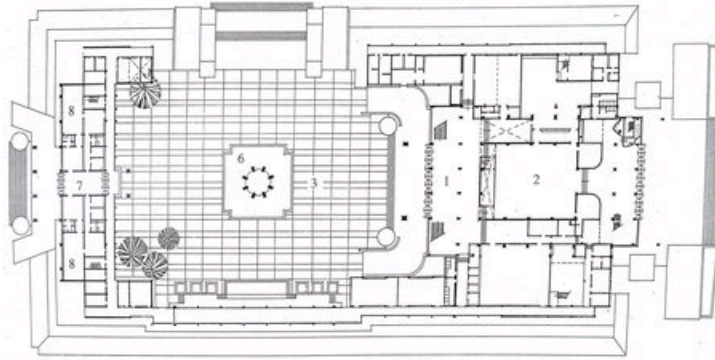
底层平面图
