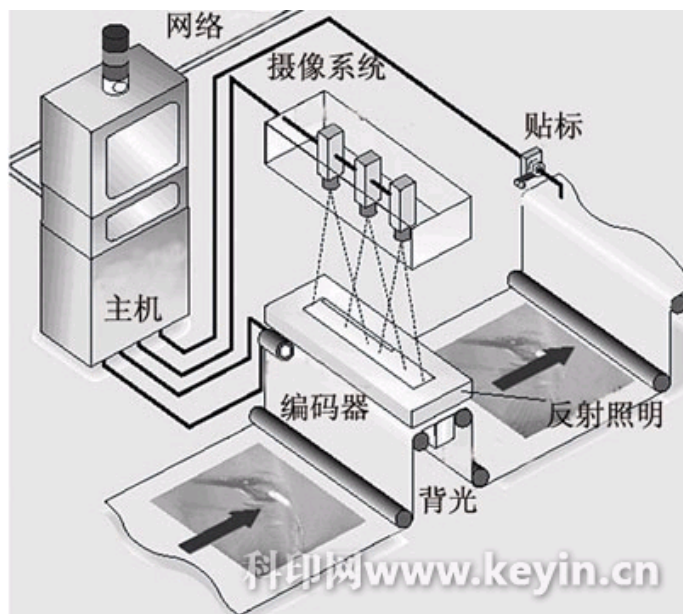
图1 印刷品质量检测系统示意图
